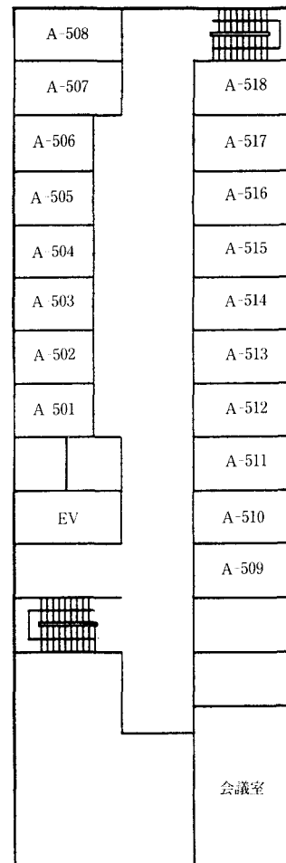
A 棟 5 階
