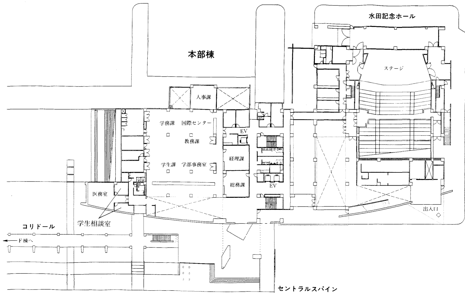
本部棟 1階
