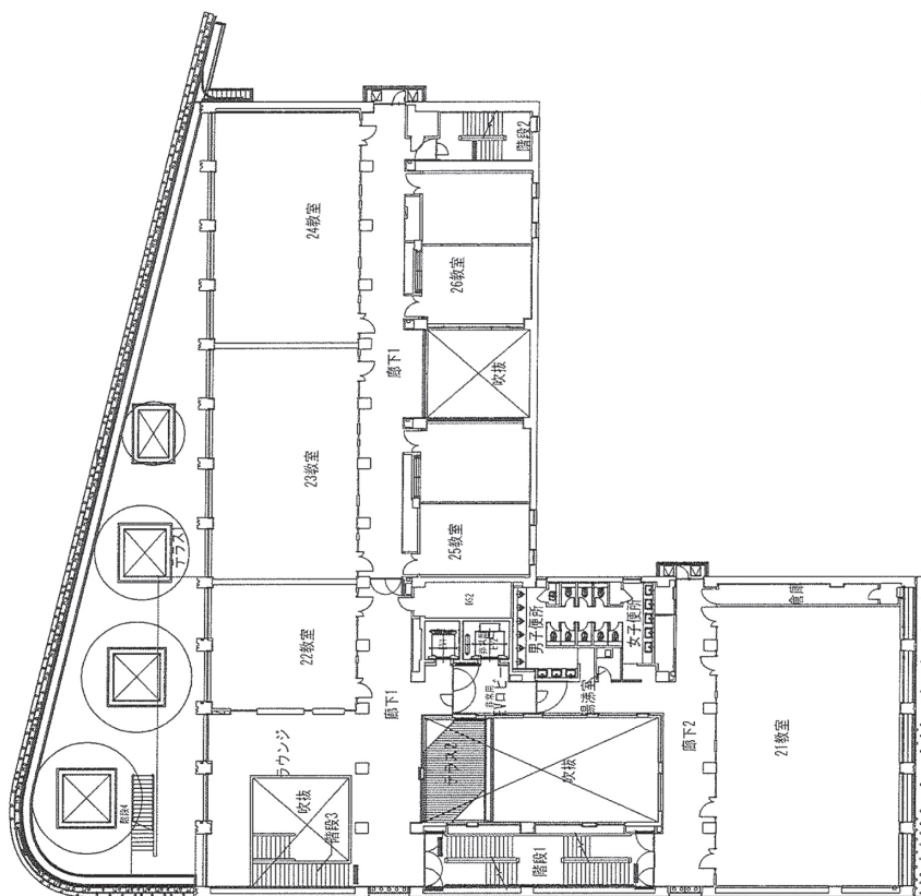
2 階
