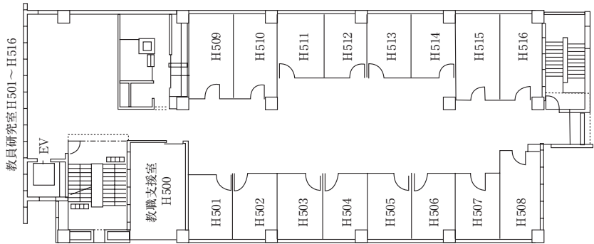
H棟 5階
